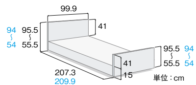
セーフティラウンドボード
